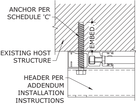
2 15 WALL MOUNT N.T.S. HORIZ SECTION
