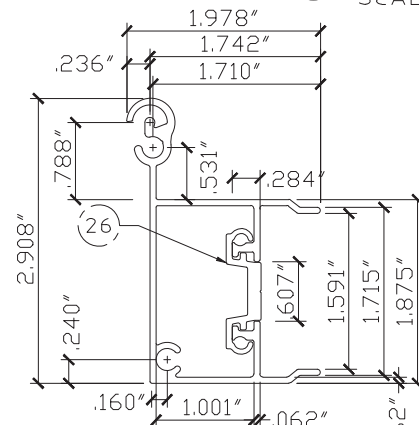
31 MALE BOX CENTER SCALE: HALF SIZE
