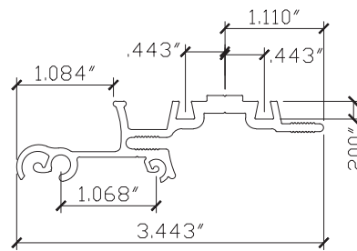
29 2003 6.8 CENTER MATE SCALE: HALF SIZE
