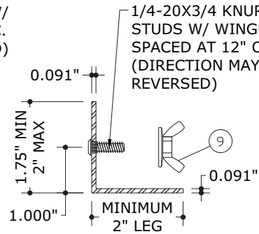
4a STUD ANGLE
