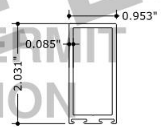
5 PQ010231 THUMB TURN HOUSING N.T.S. 6063-T6
