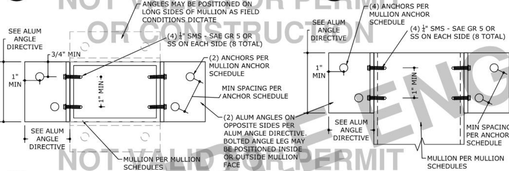
1B FACE MOUNT OPTION 1 30 N.T.S.
