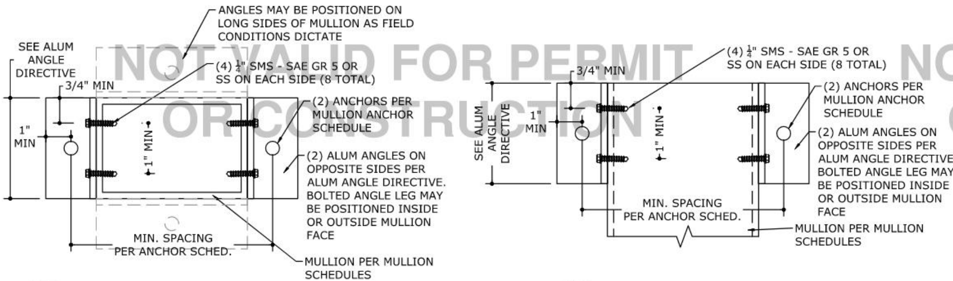
1A TRAPPED MOUNT OPTION 1 30 N.T.S.
