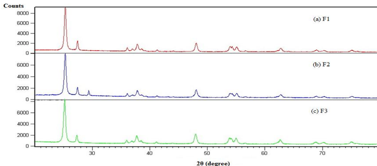
Fig. 1 XRD patterns (a) F1 film (b) F2 film (c) F3 film
