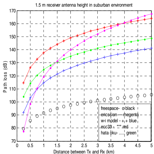
Fig 3 Pathlossfor urban area
