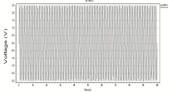
RF INPUT : SINUSODIAL 830MHz
