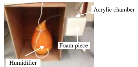
Fig. 4. Ultrasonic humidifier
