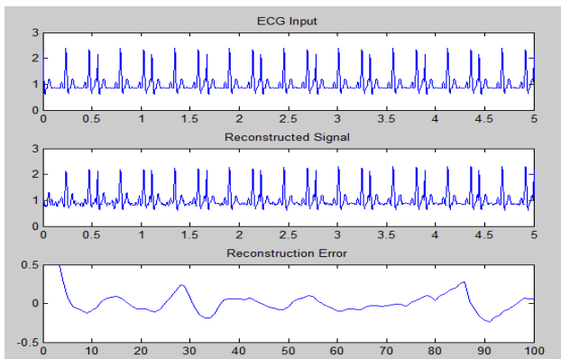
Fig. 4 DST
