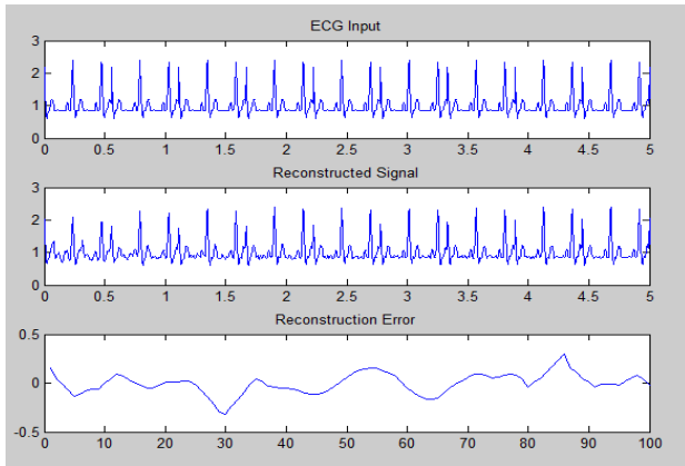
Fig. 2 DCT
