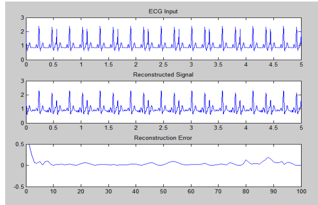
Fig. 5 FFT
