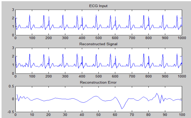
Fig. 3 DCT-II
