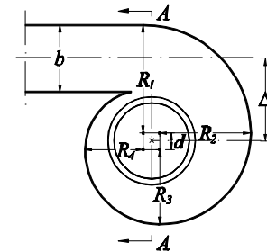
Sec. A-A
