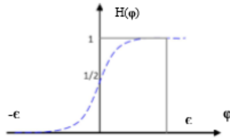
Fig. 2: Heaviside Function
