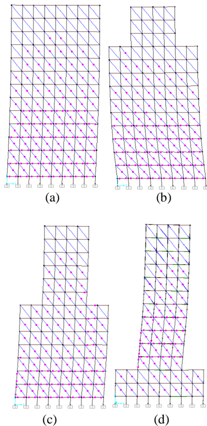
Figure 13 Hinge pattern at yielding for (a) R (b) IR3 (c) IR1 (d) IR4
